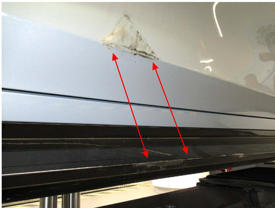
Bild 13 : Beifahrertür und Blende der Schwellerverkleidung rechts sichtbar beaufschlagt und verschrammt.
